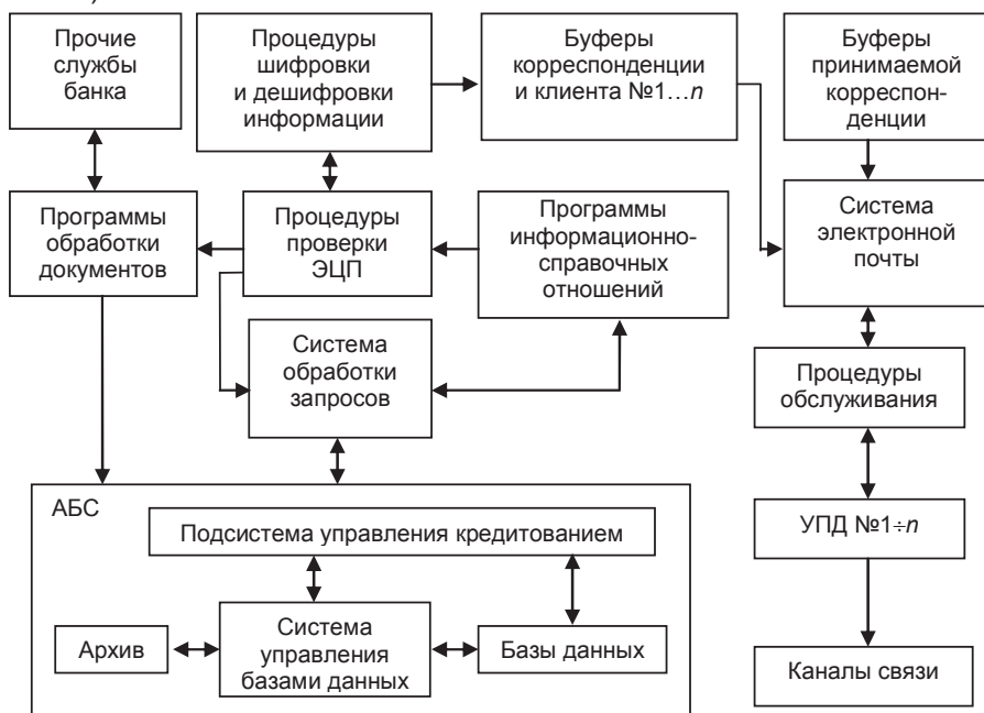
Рис. 1. Структурная схема модуля «Банк»
