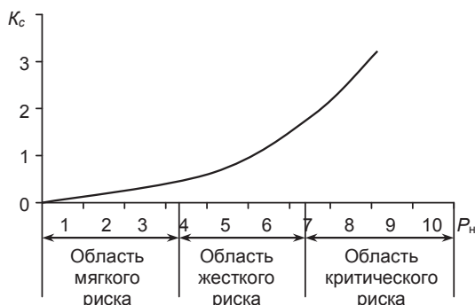
Рис. 2. Зависимость увеличения суммы выплат от вероятностного показателя невозвращения кредита
