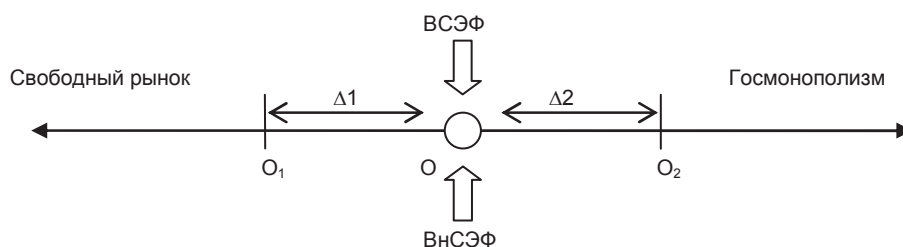
Векторная модель распределения методов госрегулирования (ВСЭФ – внешние социально-экономические факторы; ВНСЭФ – внутренние социально-экономические факторы)
